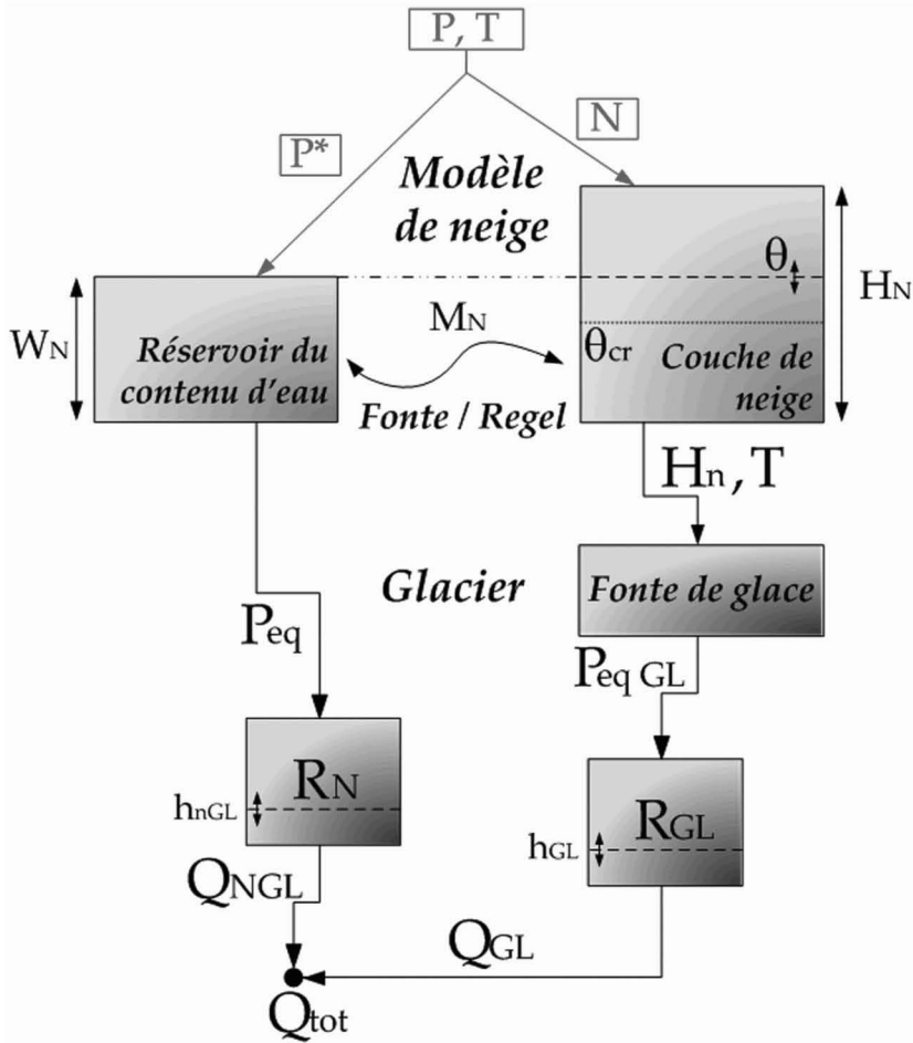
Figure 2.—Modèle hydrologique de la partie glaciaire. Données d'entrée: précipitation ( P ) et température ( T ). Données de sortie: débit glaciaire ( Q_{GL} ), débit non-glaciaire ( Q_{NGL} ) et débit total ( Q_{tot} ). P^* représente la précipitation liquide, N la précipitation solide, H_N la hauteur de neige, W_N la hauteur d'eau, \theta le contenu relatif d'eau dans le stock de neige, \theta_{cr} le contenu d'eau dans le stock de neige à partir duquel la précipitation équivalente est produite, M_N la fonte ou congélation de la neige, P_{eq} et P_{eq\ GL} la précipitation équivalente provenant de la fonte de neige ou de glace. R_N et R_{GL} concernent les réservoirs linéaires de neige et glace, et h_{nGL} et h_{GL} les niveaux d'eaux dans ces réservoirs. (figure 4.2 en couleur en annexe)
